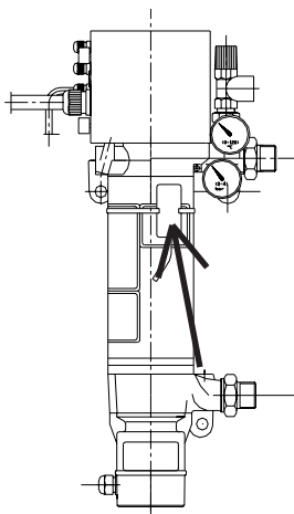
Fühlermontage am Mantelrohr: Der Fühler muß so hoch wie möglich montiert werden, auf guten Kontakt ist zu achten!
