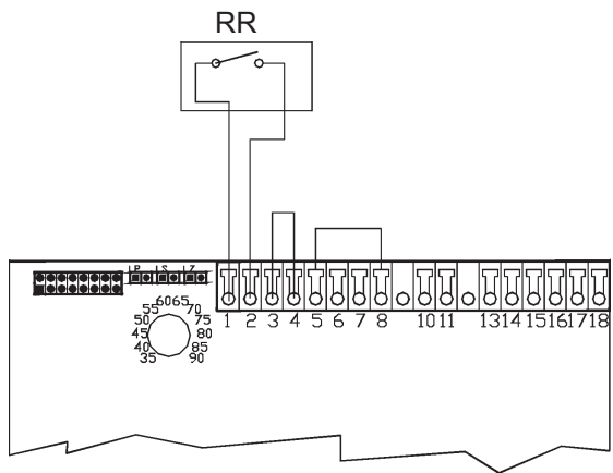
Anschlußschema für Rundsteueranlage wenn nur ein oder zwei Heizregister über die Rundsteueranlage geschaltet werden
