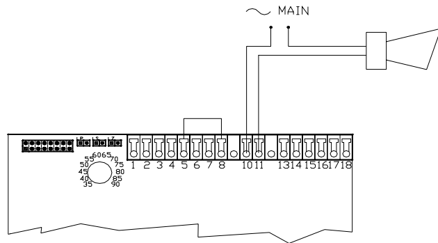
Anschlußschema Ansteuerung einer Hupe mit dem Alarmausgang
