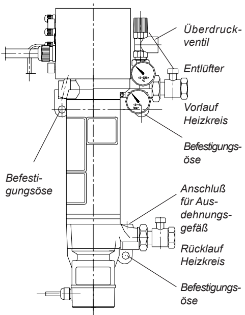
Anschluß Baureihe EPR
