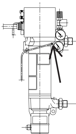
Fühlermontage in der Tauchhülse: Der Fühler wird in die Bohrung am Kopfteil der Elektroheizpumpe eingeschoben. Zur Verbesserung des thermischen Kontakts sollte Wärmeleitpaste verwendet werden!
