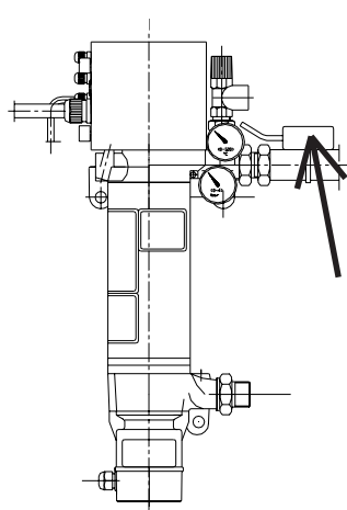
Fühlermontage am Vorlauf: Der Fühler muß vor dem ersten Abgang liegen und muß metallischen Kontakt haben.
