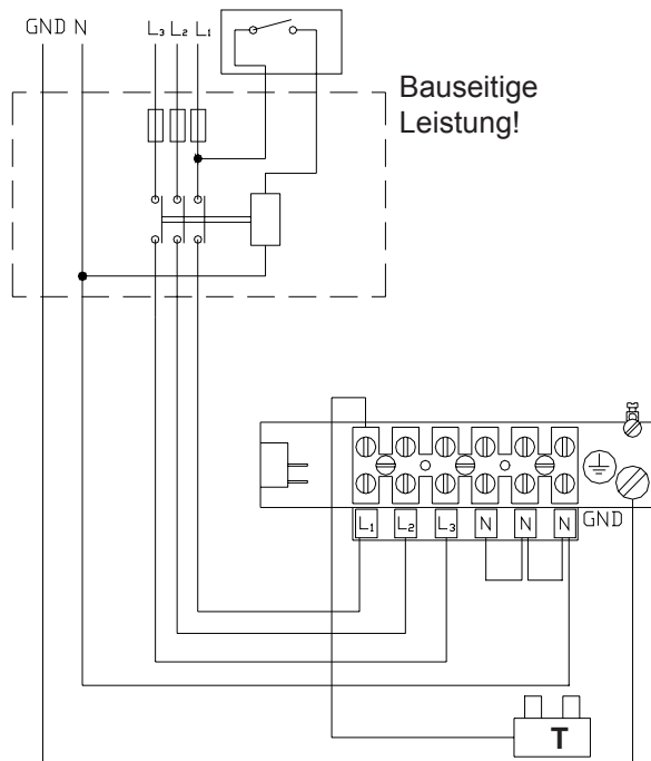
Anschlußschema für Rundsteueranlage wenn die gesamte Heizleistung geschaltet werden soll.
