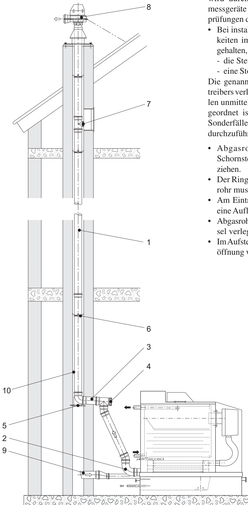
Bild 2-3: VERITHERM-Brennwertkessel mit herkömmlichem Abgassystem. Das Abgasgebläse ist am Ende der Abgasleitung installiert, das System steht unter Unterdruck!
