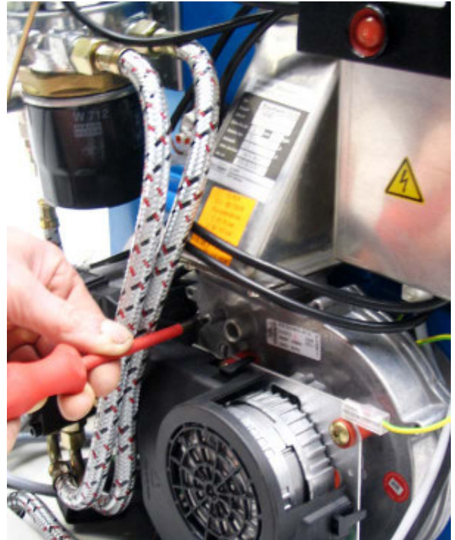
Bild 3-5: Messung der Verbrennungsluft (CO 2 , Temperatur u.ä.).
