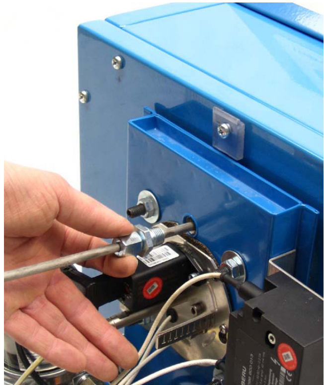
Bild 2-9: Messstutzen für die CO 2 - und Unterdruck-Messung.
