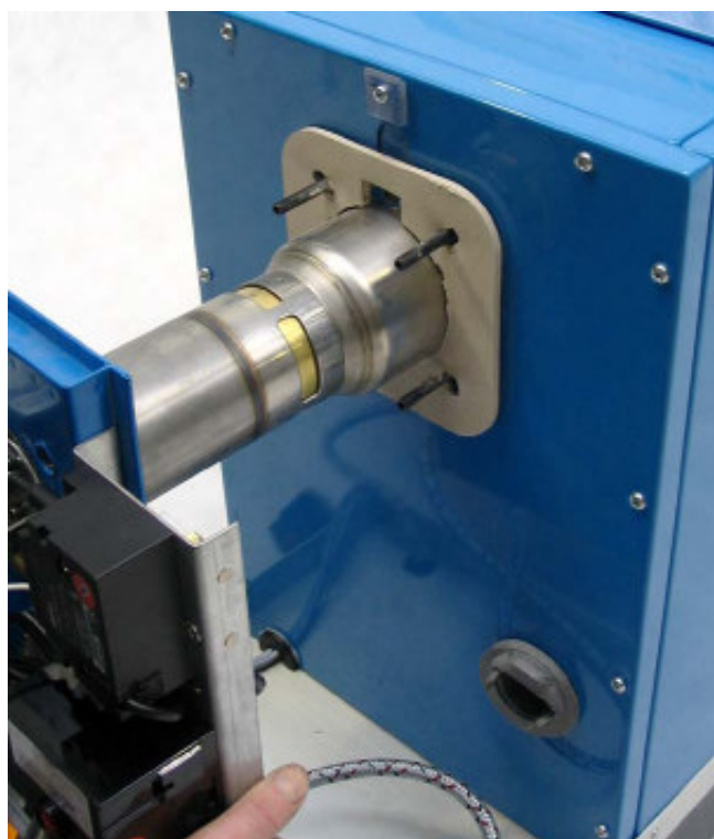
Bild 3-8: Brenner mit Glührohr vorsichtig aus der Brennkammer herausziehen.
