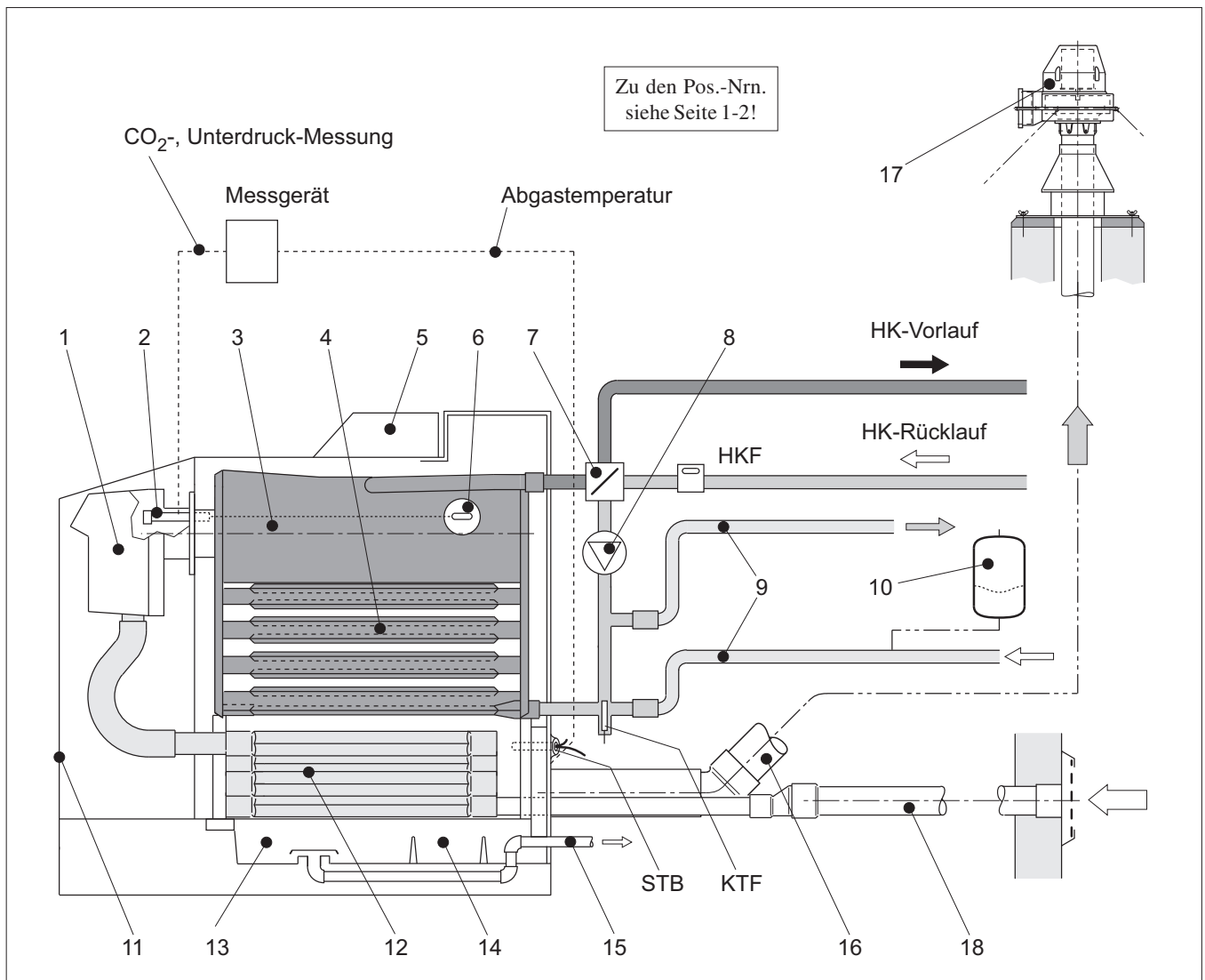
Bild 2-1: Schema der Heizungsanlage
